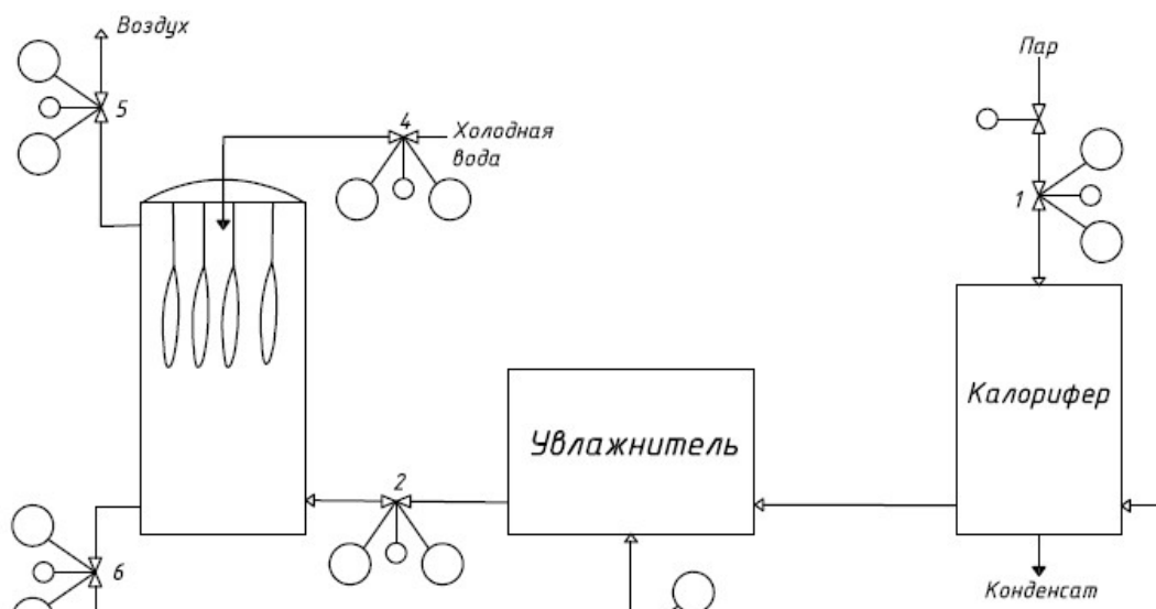
Рисунок 4 – Технологическая схема
