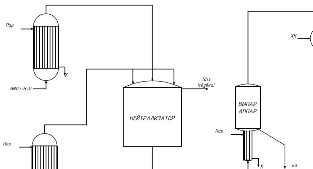
Рисунок 3 – Технологическая схема
