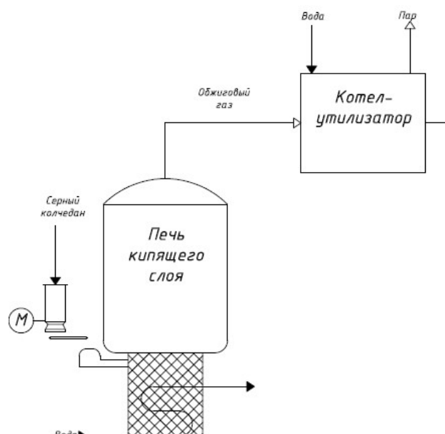
Рисунок 1 – Технологическая схема
